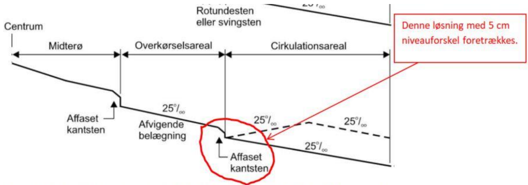
Figur 7.7 Tværsnit af midterø og overkørselsareal med eksempler på begrænsning. Hvis kantbegrænsningen ikke udføres med hvide sten, afmærkes der med en kantlinje.
